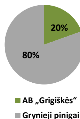
Portfelio sudėtis (2011.04.22)
